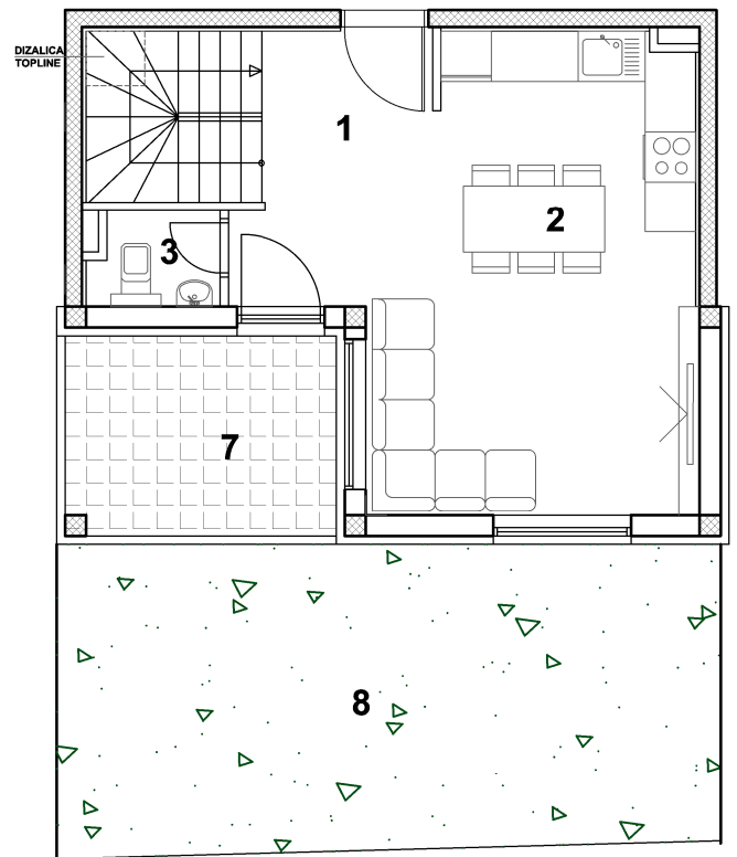
1 ETAŽA - PRIZEMLJE
