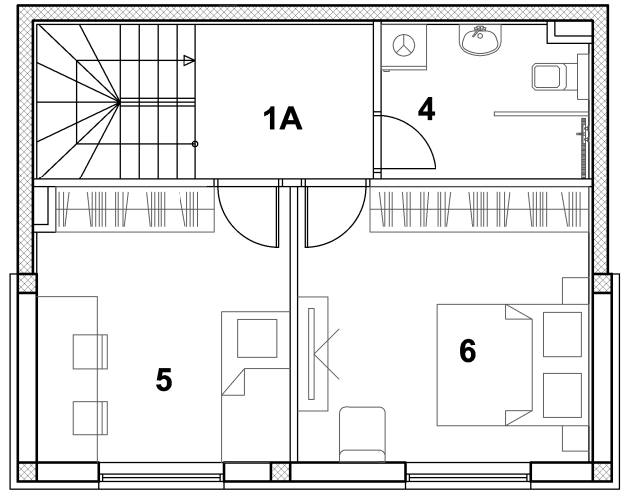
2 ETAŽA - 1. KAT
